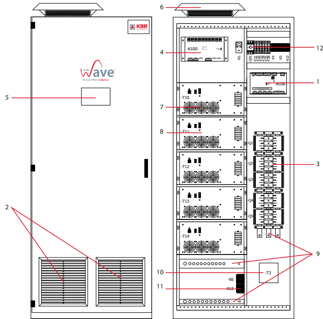
A | Standschrank
